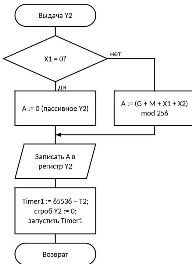
Рис. 12. Схема алгоритма: Расчёт и выдача сигнала Y2
