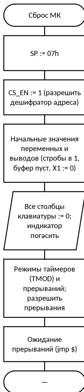
Рис. 1. Схема алгоритма: Инициализация МПС и основная программа
