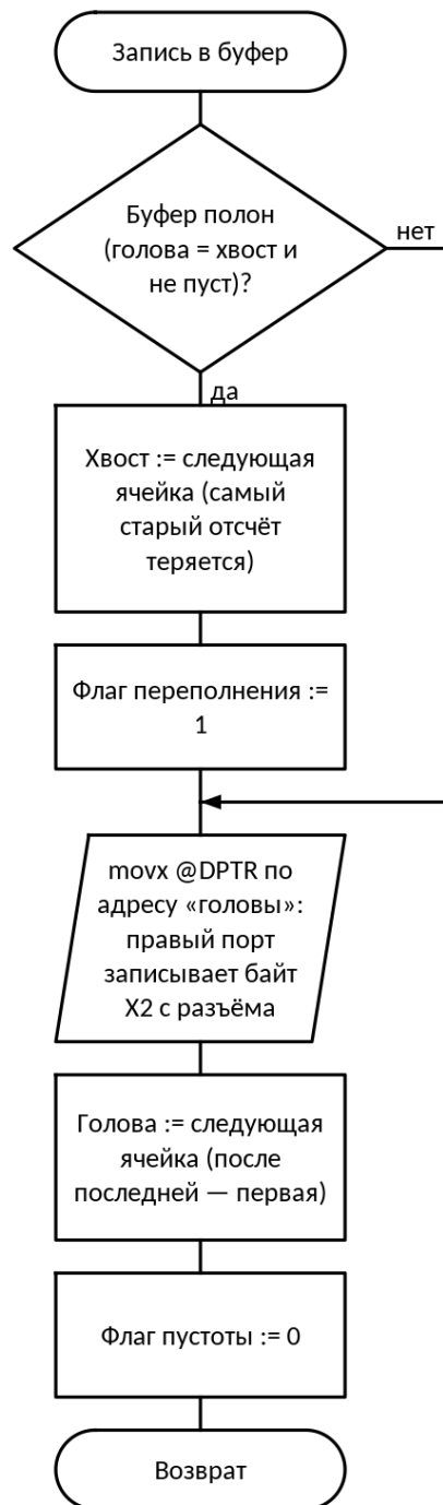
Рис. 5. Схема алгоритма: Запись отсчёта в кольцевой буфер
