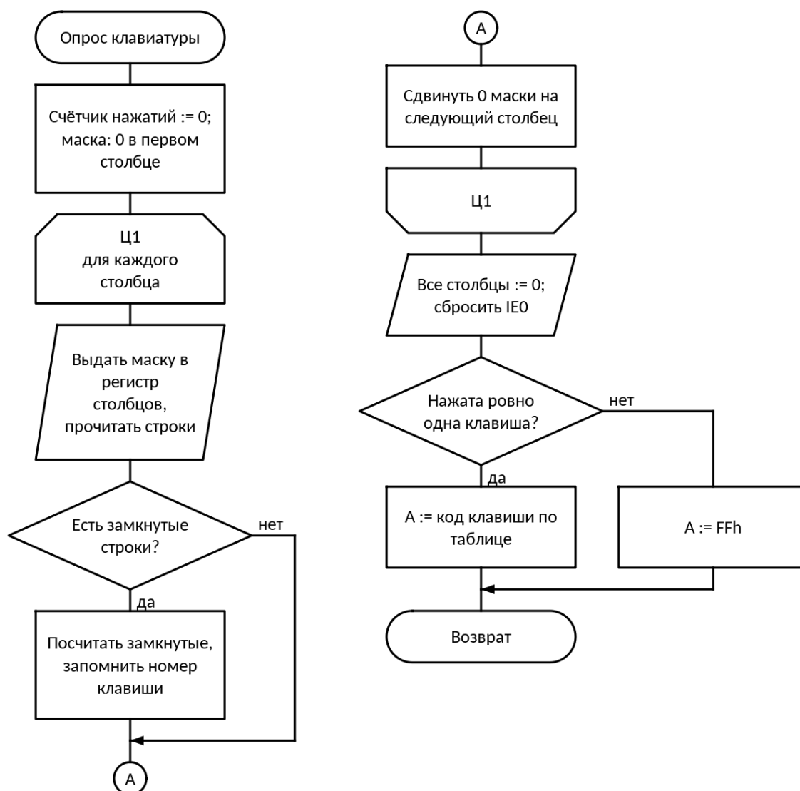
Рис. 3. Схема алгоритма: Опрос клавиатуры (обработчик INT0)
